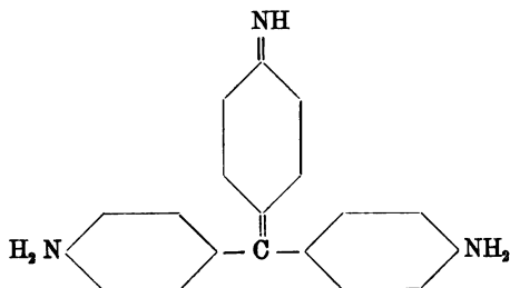
Diaminofuchsonimin.
